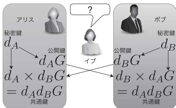
図 20: 楕円曲線 Diffie-Hellman
