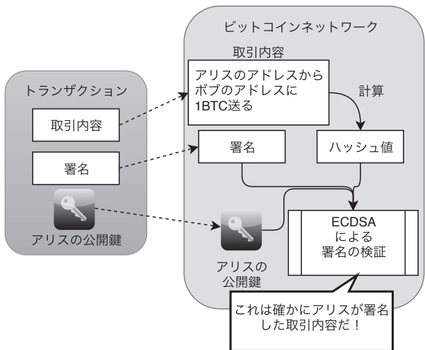
図 7: トランザクションの検証
