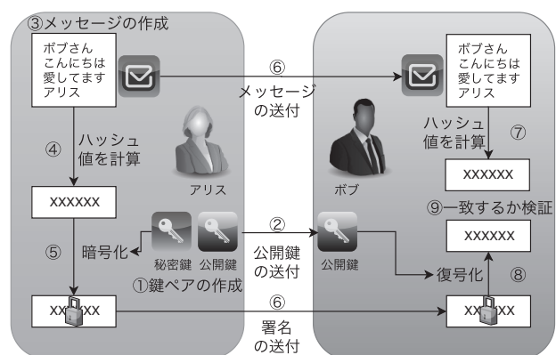
図 5: RSA を用いたデジタル署名
