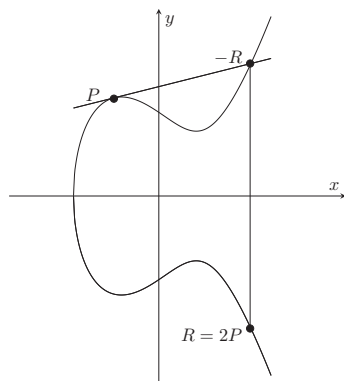
図 10: 楕円曲線上の加法 ( P = Q の場合)
