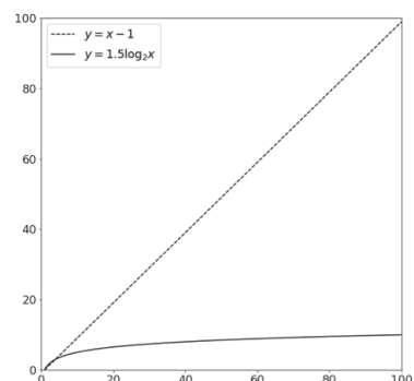
図 17: 計算量の比較 (100 まで)
