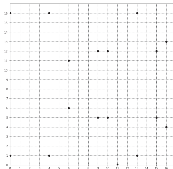
図 11: \mathbb{F}_{17} 上での楕円曲線 y^2 = x^3 + x + 1
