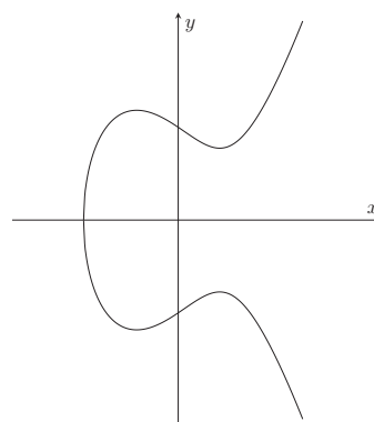
図 8: 楕円曲線
