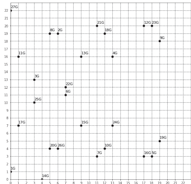
図 14: \mathbb{F}_{23} 上での楕円曲線 y^2 = x^3 + x + 1
