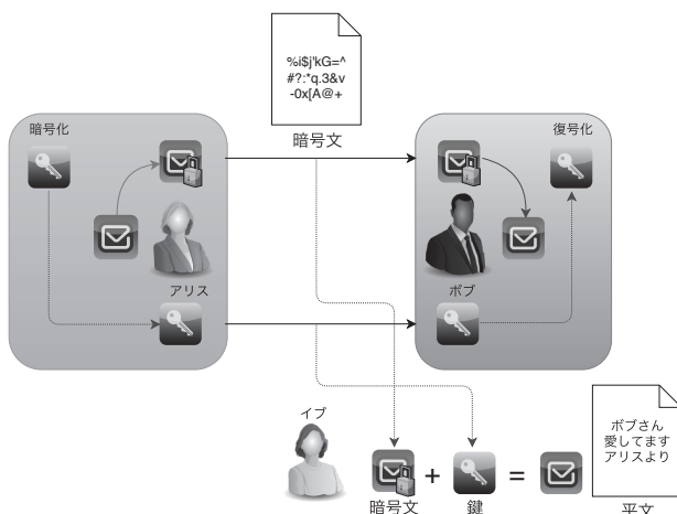
図 3: 鍵配送問題
