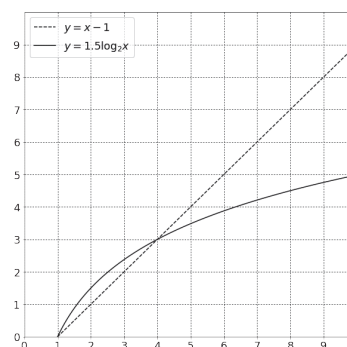
図 16: 計算量の比較 (10 まで)
